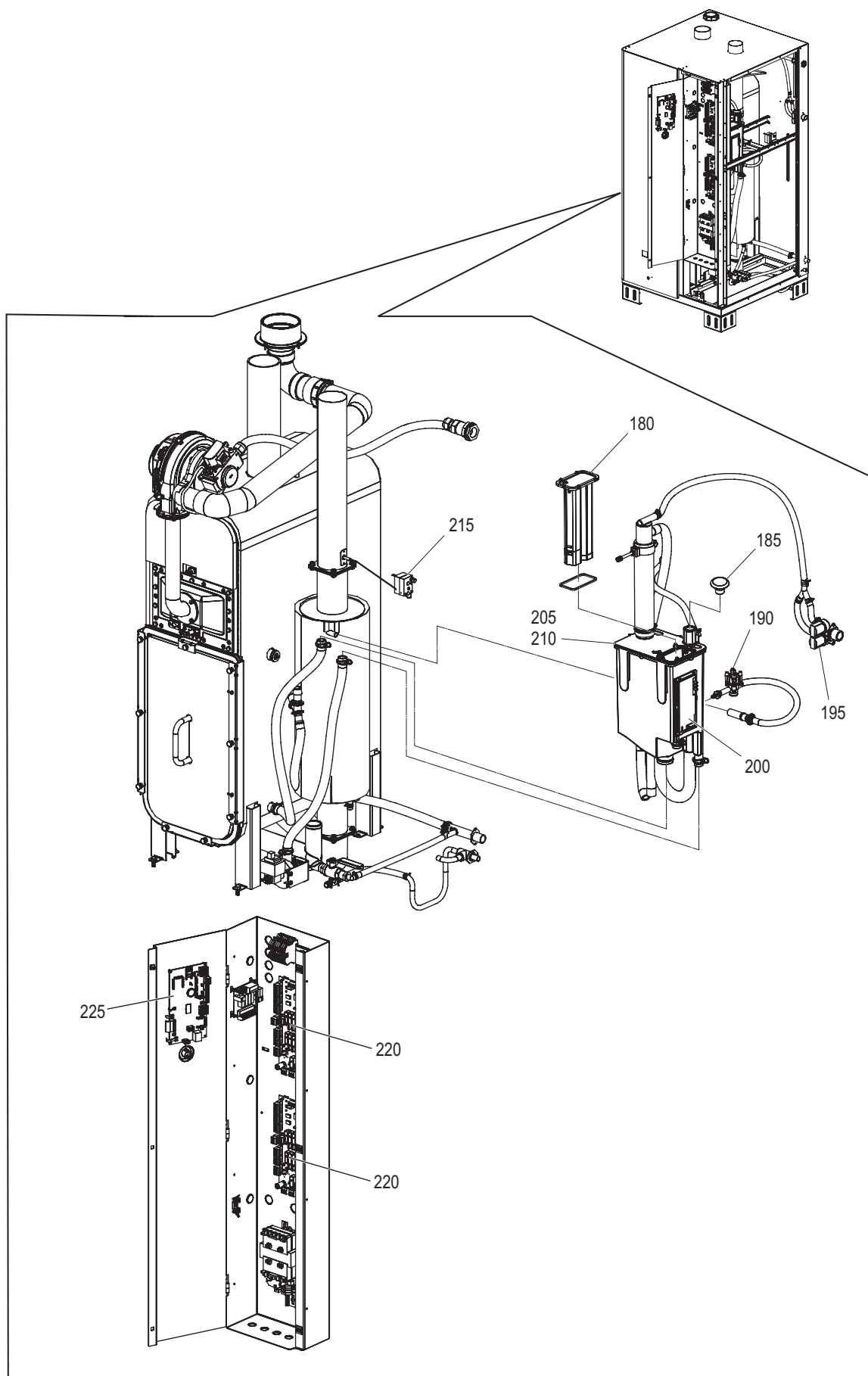
Figuur 2: Condair GS-luchtbevochtiger, water- en elektrische leidingen
