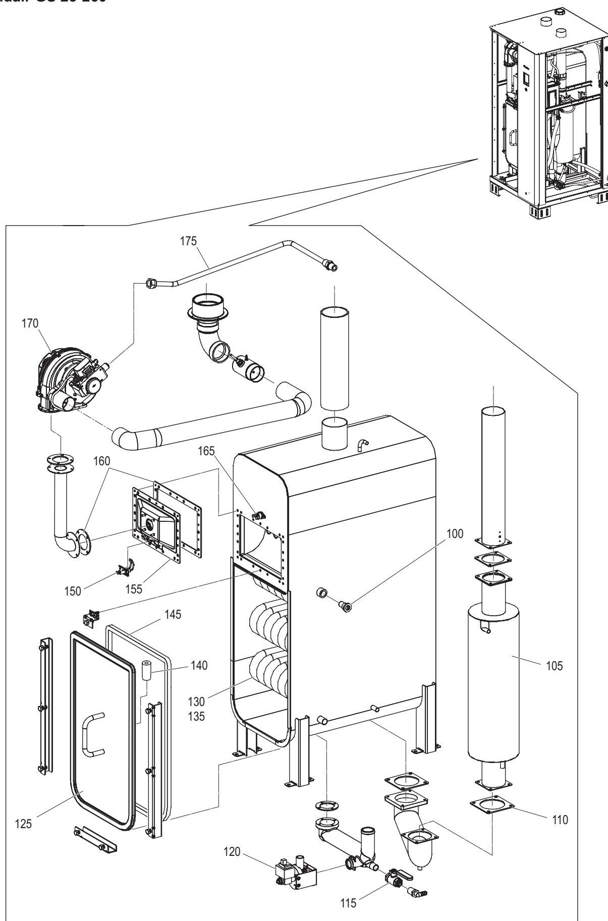
Figuur 1: Condair GS-luchtbevochtiger, warmtewisselaar en ventilator
