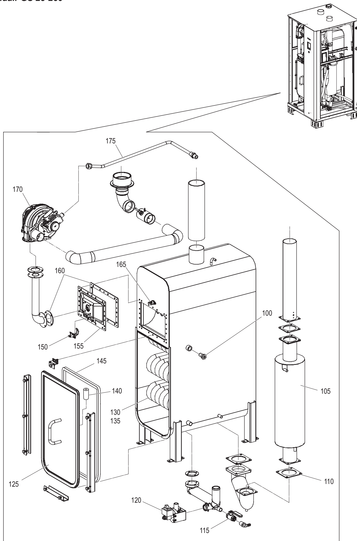
Figuur 1: Condair GS-luchtbevochtiger, warmtewisselaar en ventilator, vervolgd ...
